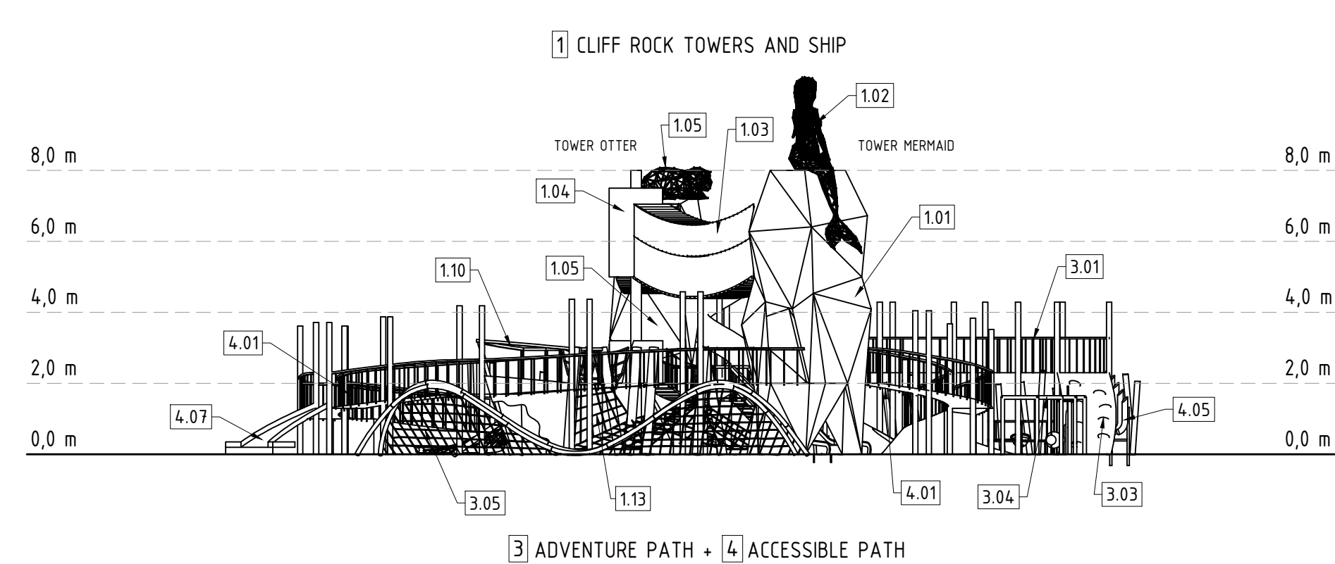
ELEVATION D1
